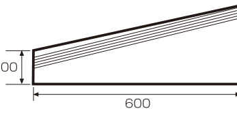
歩車道ブロックA乗入6型(右)(A-6)
