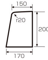
歩車道ブロックA乗入4型(右)(A-4)
