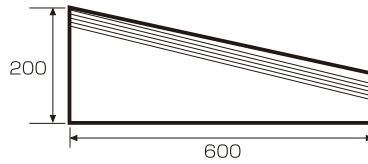
歩車道ブロックA乗入6型(右)(A-6)
