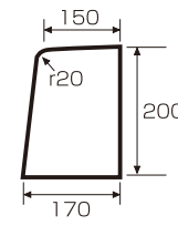
歩車道ブロックA乗入6型(右)(A-6)
