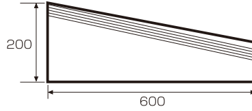
歩車道ブロックA乗入4型(右)(A-4)
