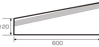
歩車道ブロックA乗入5型(左)(A-5)
