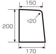
歩車道ブロックA乗入5型(左)(A-5)
